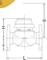
Esquema de dimensiones Esquema de dimensões
